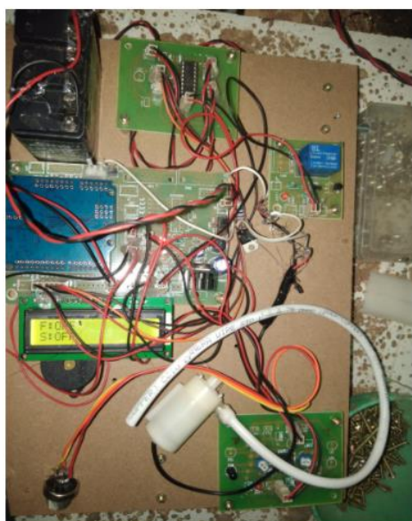
Fig.4.1. Hardware circuit.
